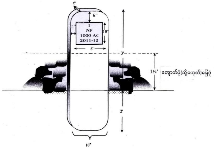
သစ်သားဘုတ်တိုင်(ကျောက်ပုံ)
