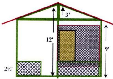
ပင်မတဲ ဆောက်လုပ်ရန်ပုံစံ (အရှေ့ဘက်မှမြင်ရပုံ)
