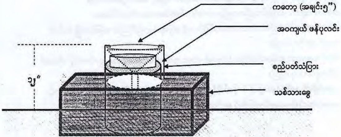
သစ်သားခွေ (၁၅' x ၁၅' x ၁')
