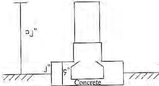
မိုးရေချိန်တိုင်းကိရိယာတပ်ဆင်ထားပုံ
