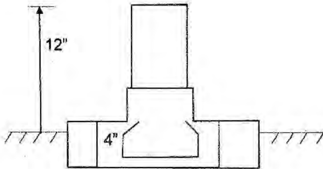
မိုးရေချိန်တိုင်းကိရိယာတစ်ခု တပ်ဆင်ထားပုံ
